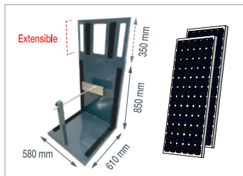
SOLAR PANEL PLATFORM PLATTFORM FÜR SOLARMODULE
